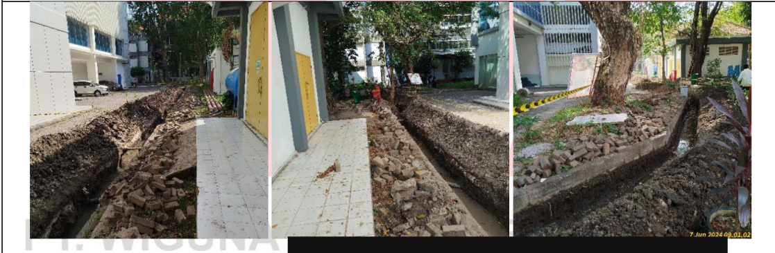
7 Juni 2024 - Pekerjaan galian U-Ditch
