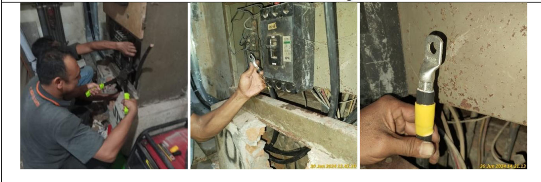
30 Juni 2024 - Terminasi kabel Gedung Statistik
