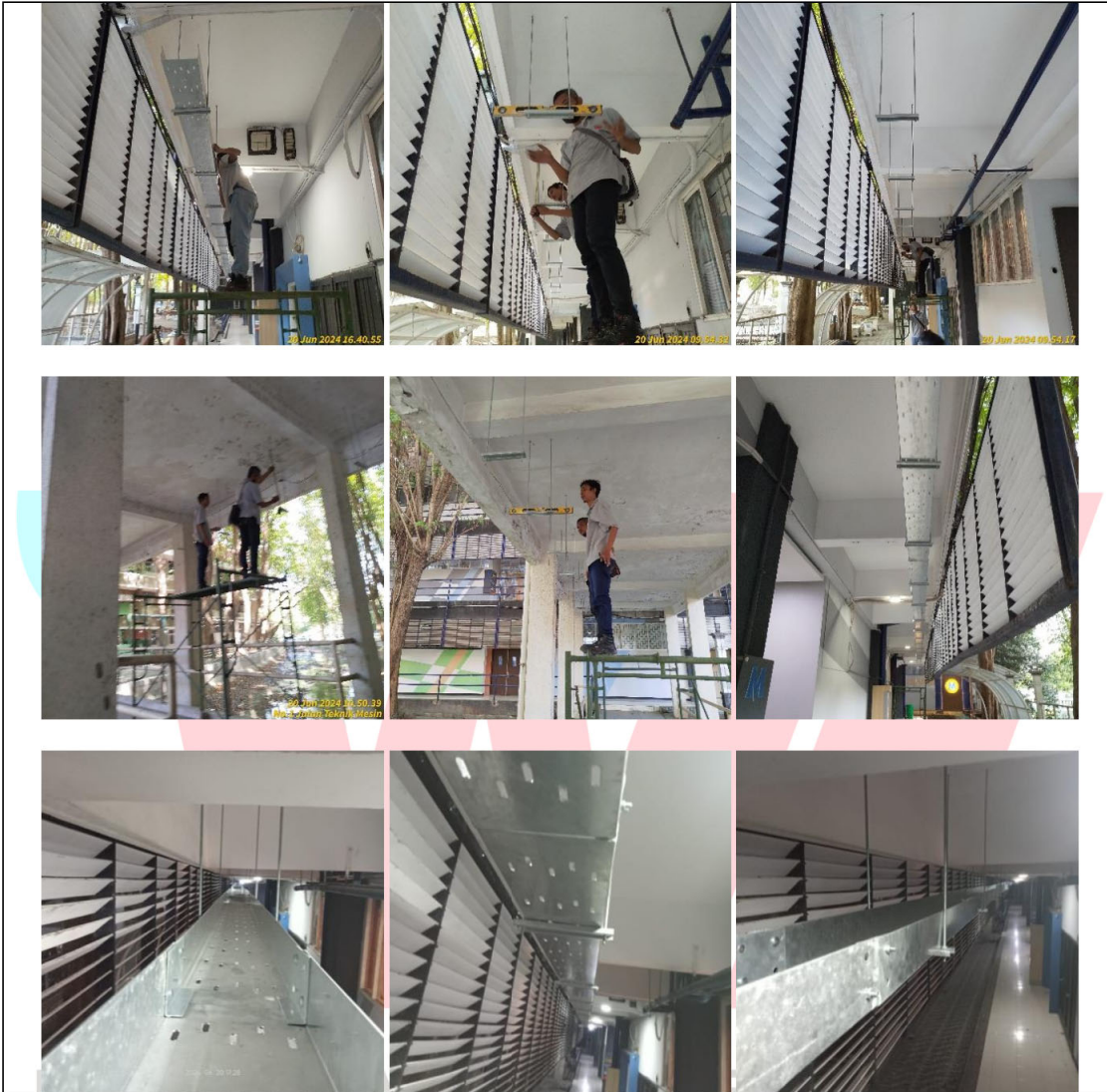
21 Juni 2024 – Pemasangan kabel tray
