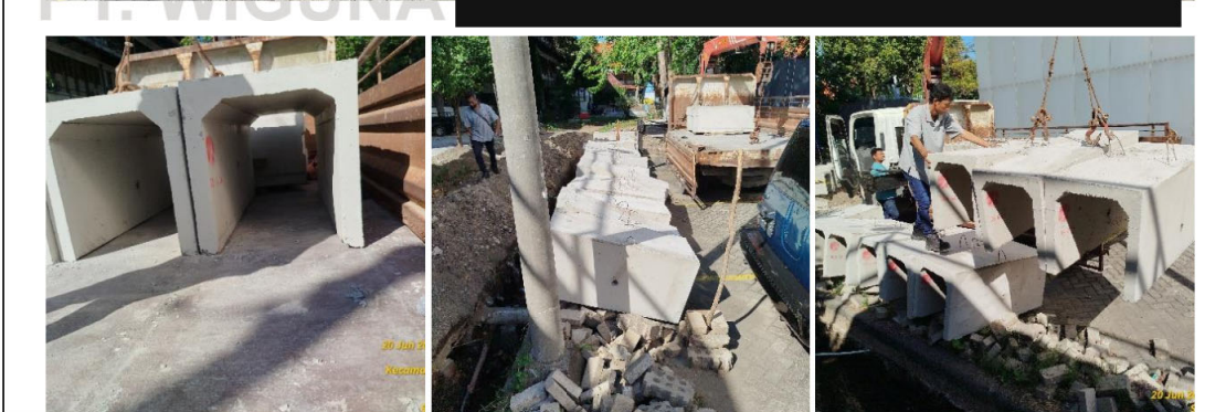
21 Juni 2024 – U-Ditch on site & pekerjaan pemasangan U-Ditch
