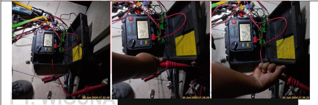
30 Juni 2024 - Insulation test sesudah terminasi kabel 95mm
